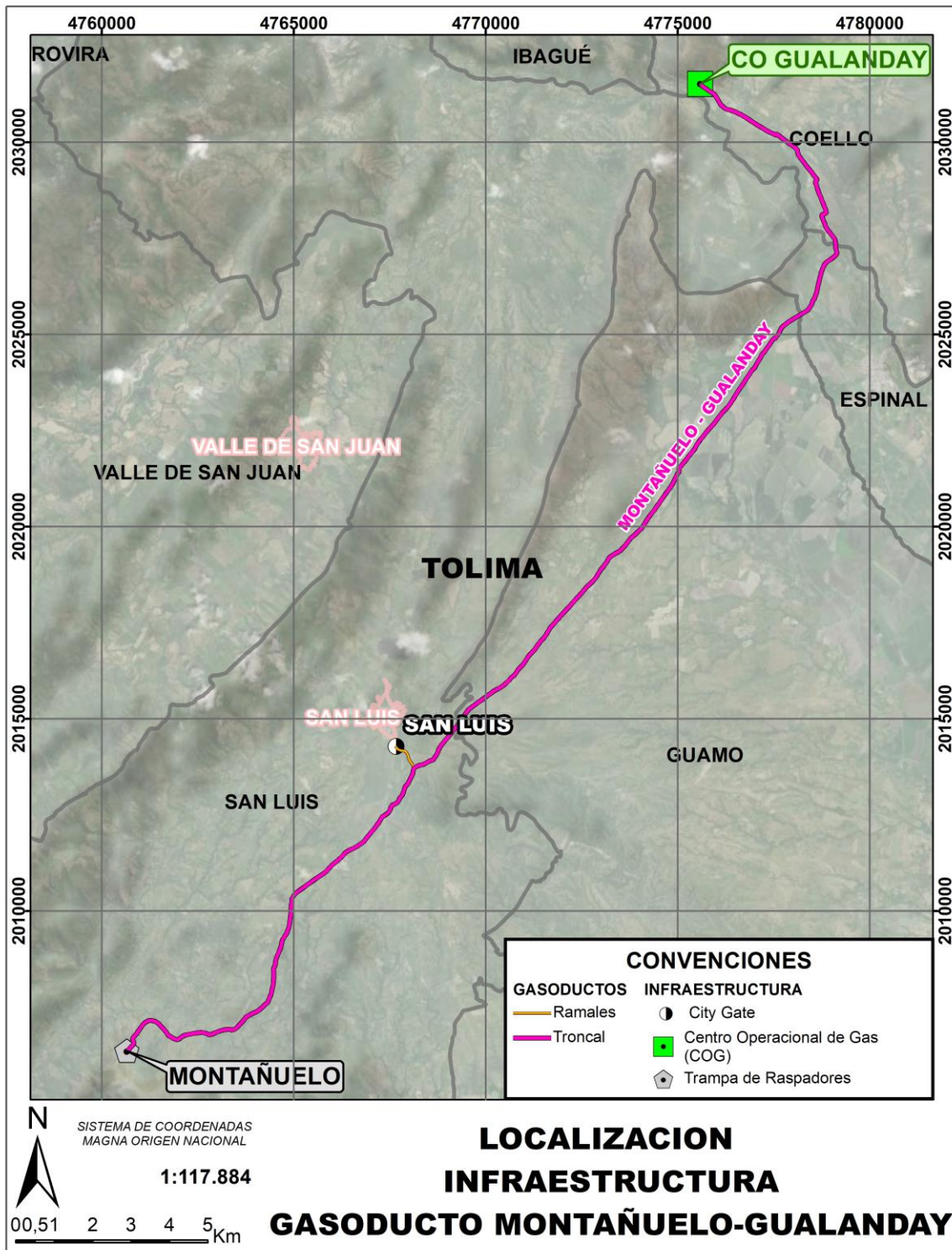
Figura 3. Localización infraestructura Gasoducto Montañuelo - Gualanday
