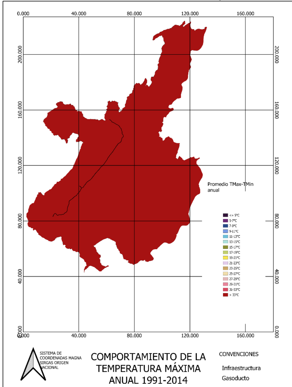
Figura 7. Comportamiento de la temperatura máxima anual del periodo 1991-2014 en la zona del Gasoducto Montañuelo – Gualanday
