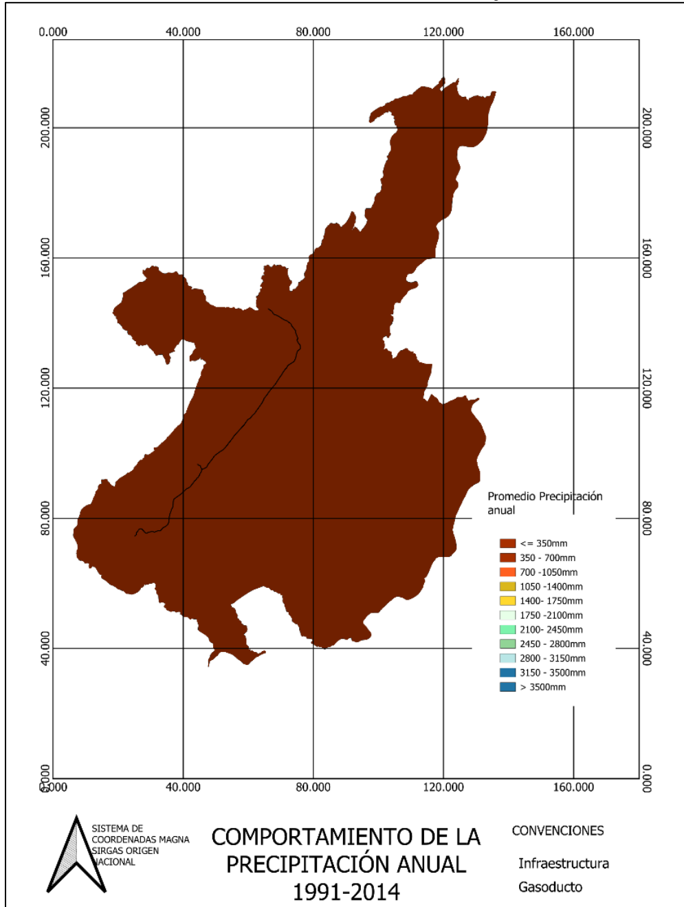
Figura 6. Comportamiento de la precipitación anual del periodo 1991-2014 en la zona del Gasoducto Montañuelo - Gualanday
