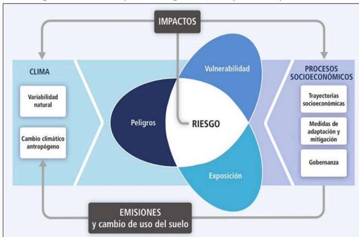
Figura 2. Marco Conceptual de riesgos climáticos presentado por el IPCC
