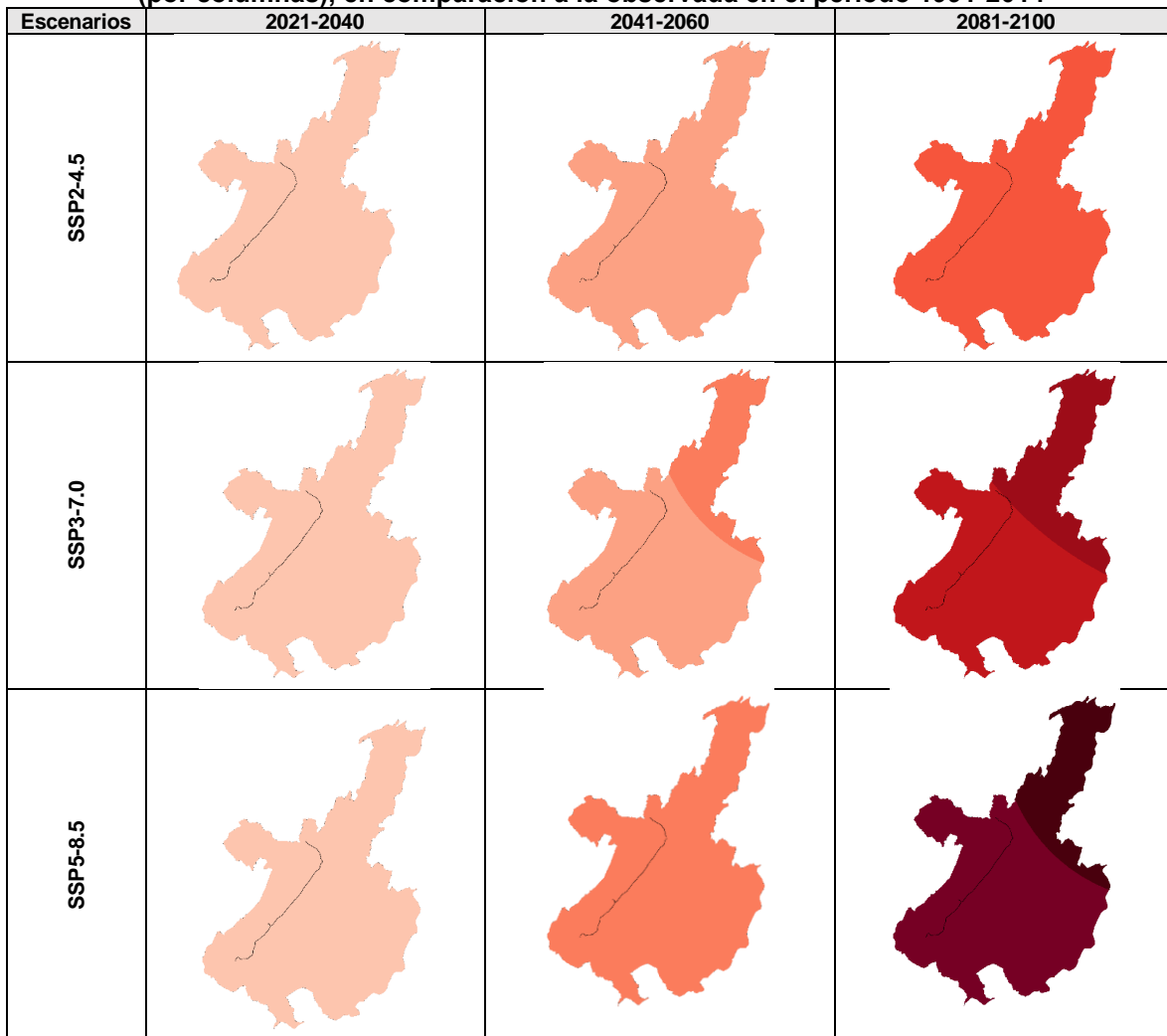
Figura 10. Aumento (°C) de la temperatura máxima anual bajo los escenarios SSP2-4.5, SSP3-7.0 y SSP5-8.5 (por filas), para los periodos futuros 2021-2040, 2041-2060 y 2081-2100 (por columnas), en comparación a la observada en el periodo 1991-2014
