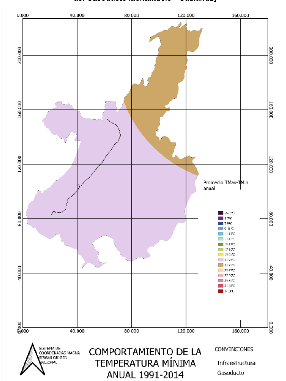
Figura 8. Comportamiento de la temperatura mínima anual del periodo 1991-2014 en la zona del Gasoducto Montañuelo - Gualanday
