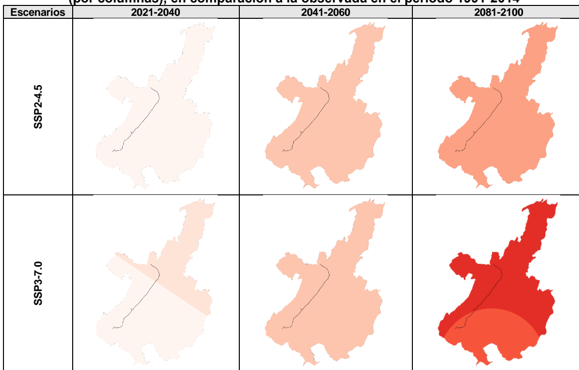
Figura 11. Aumento (°C) de la temperatura mínima anual bajo los escenarios SSP2-4.5, SSP3-7.0 y SSP5-8.5 (por filas), para los periodos futuros 2021-2040, 2041-2060 y 2081-2100 (por columnas), en comparación a la observada en el periodo 1991-2014
