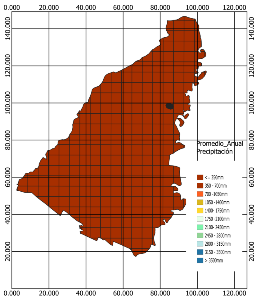
Figura 6. Comportamiento de la precipitación anual del periodo 1991-2014 en la zona del Estación de Compresión de Gas La Sabana
