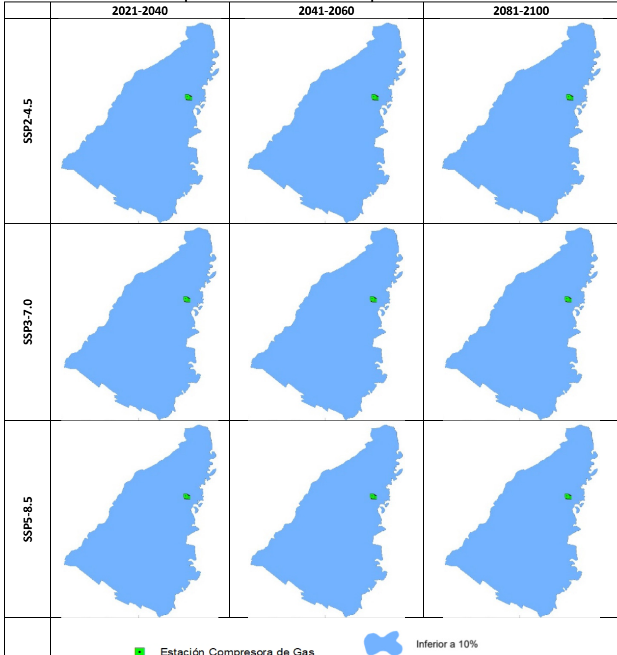
Figura 9. Cambio porcentual (%) de la precipitación anual bajo los escenarios SSP2-4.5, SSP3-7.0 y SSP5-8.5 (por filas), para los periodos futuros 2021-2040, 2041-2060 y 2081-2100 (por columnas), en comparación a la observada en el periodo 1991-2014
