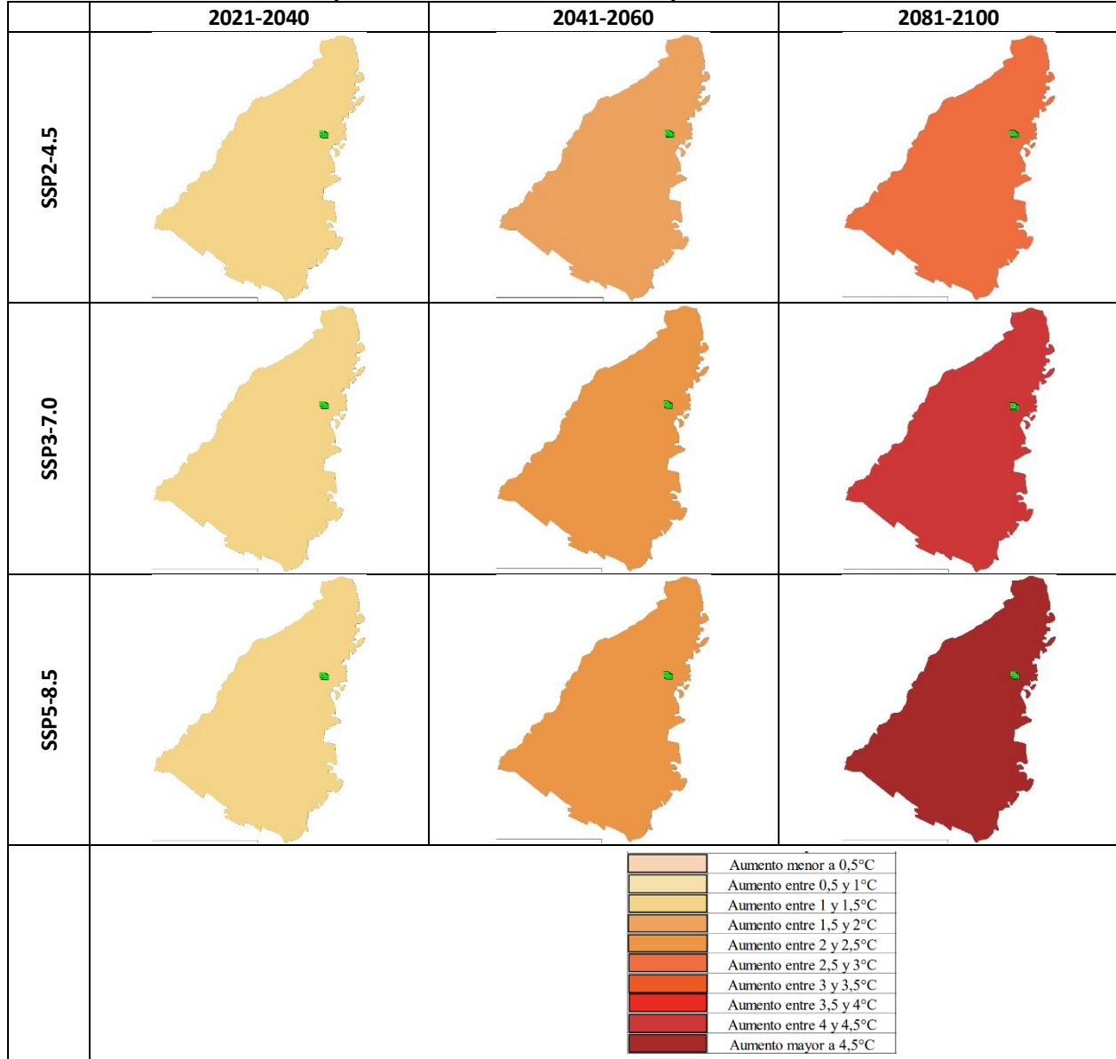
Figura 10. Aumento (°C) de la temperatura máxima anual bajo los escenarios SSP2-4.5, SSP3-7.0 y SSP5- 8.5 (por filas), para los periodos futuros 2021-2040, 2041-2060 y 2081-2100 (por columnas), en comparación a la observada en el periodo 1991-2014
