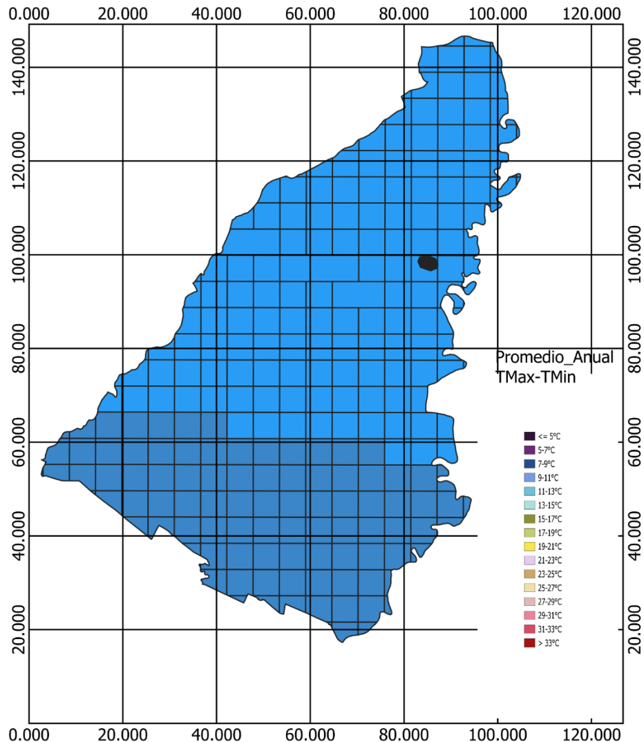
Figura 8. Comportamiento de la temperatura mínima anual del periodo 1991-2014 en la zona del Estación de Compresión de Gas La Sabana
